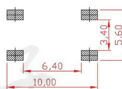
PCB. 焊接图
