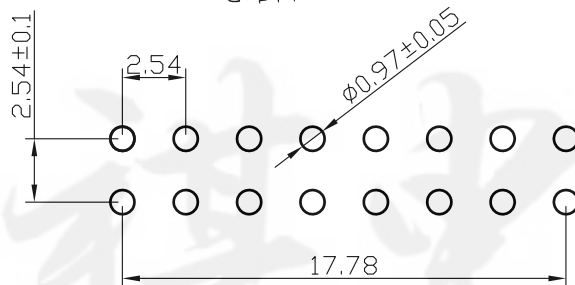
PCB开孔
