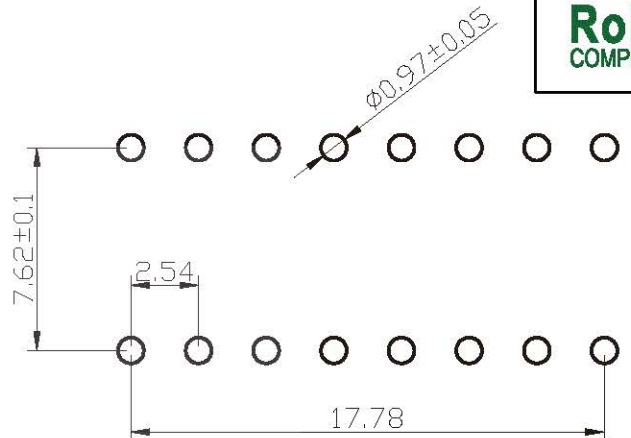
PCB开孔
