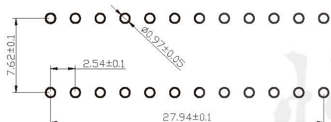
PCB开孔
