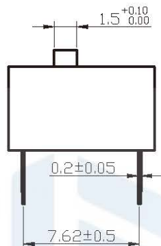
高推钮 (E)
