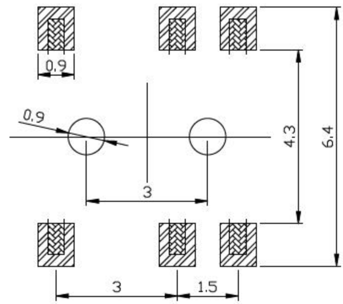
安装图 (PCB LAYOUT PLAN)
