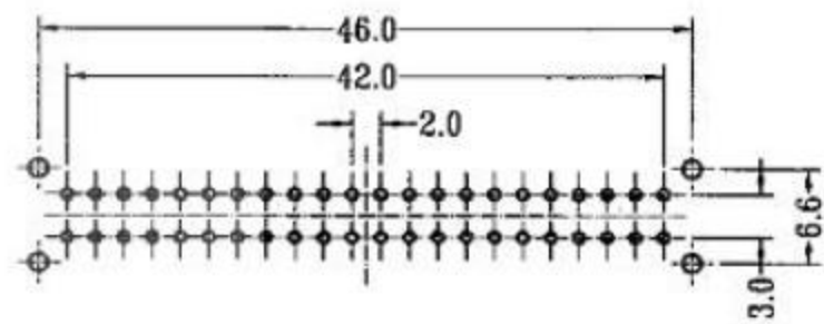
P.C.B LAYOUT
