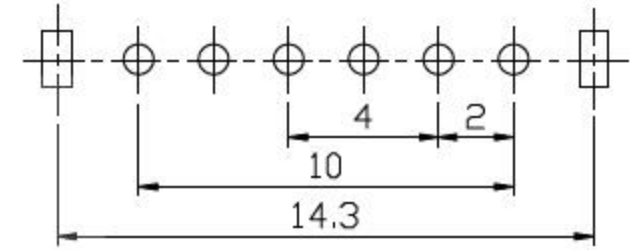
P.C.B LAYOUT
