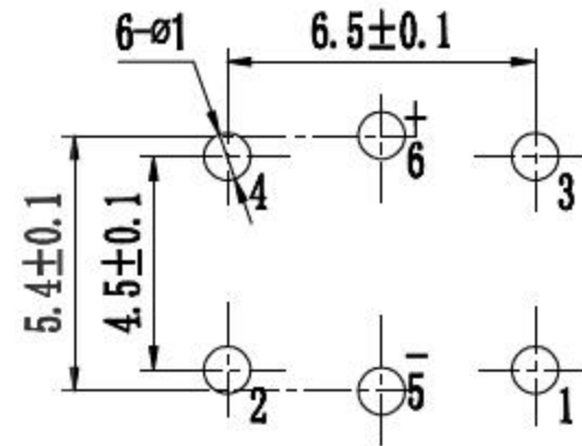
元件面孔位图
