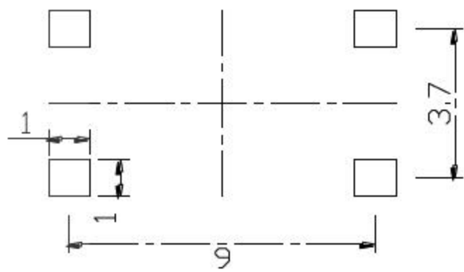
PCB. 焊接图
