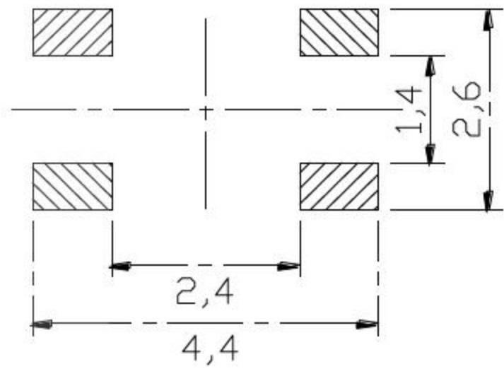
PCB. 焊接图
