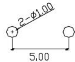
PCB. 焊接图
