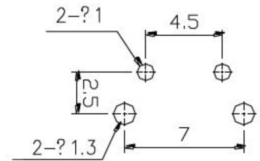
PCB. 焊接图
