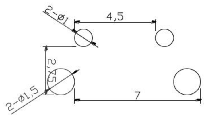
PCB. 焊接图
