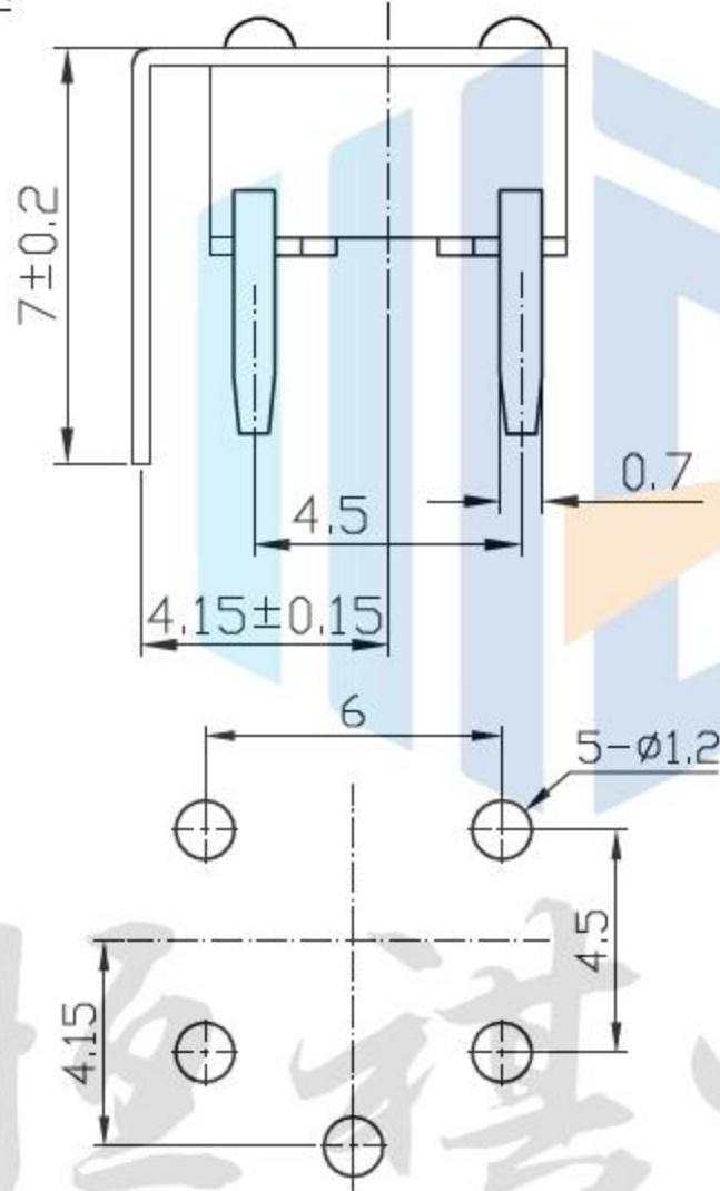
PCB线路板安装图(±0.1)
