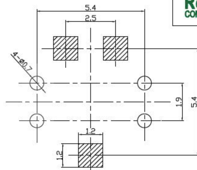
安装尺寸图
