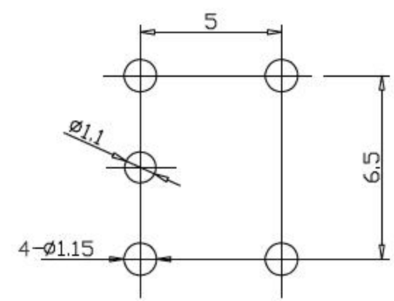
安装尺寸
