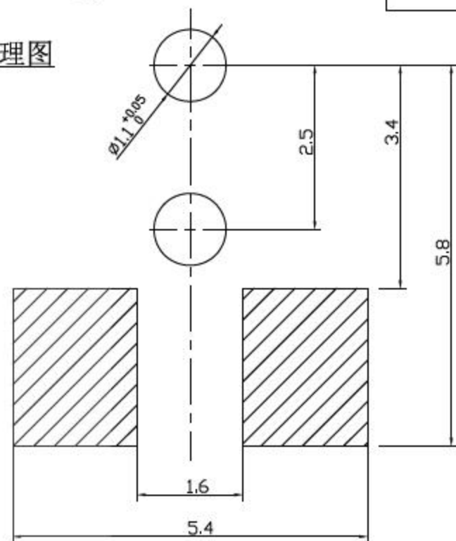
安装位置图
