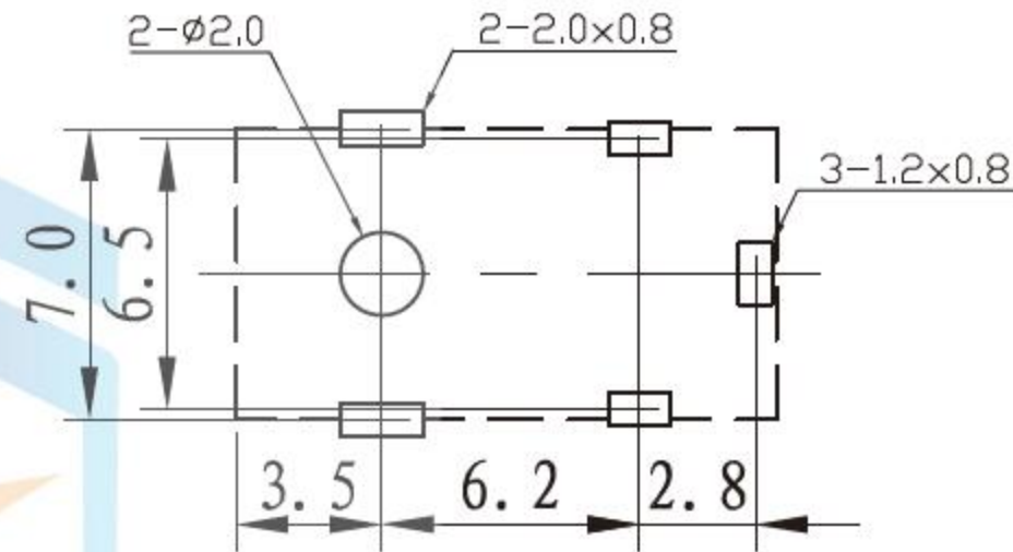
线路板安装尺寸示意图
