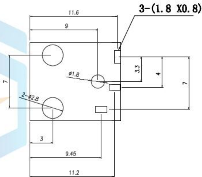
线路板安装尺寸示意图
