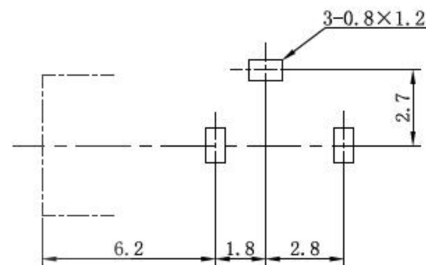
印制线路板开孔尺寸
